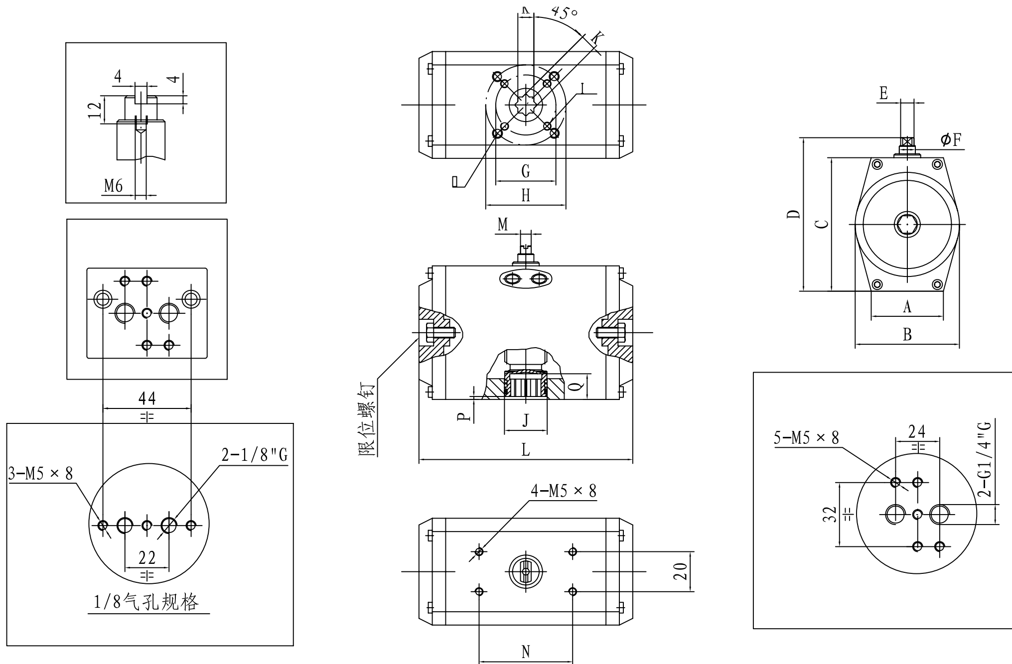
GT外形及连接尺寸
