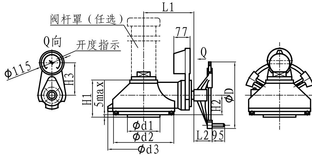
BA-S (带开度指示及微动开关) 外形尺寸
