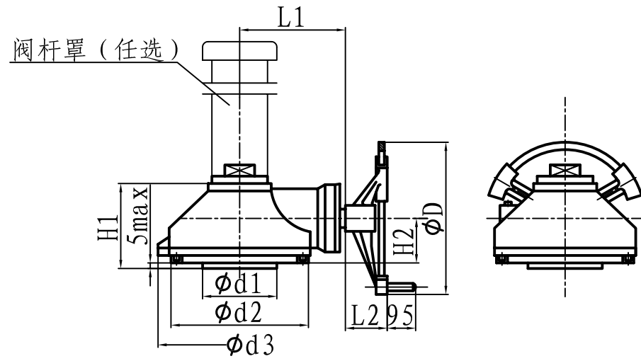
BA-P (带开度指示) 外形尺寸
