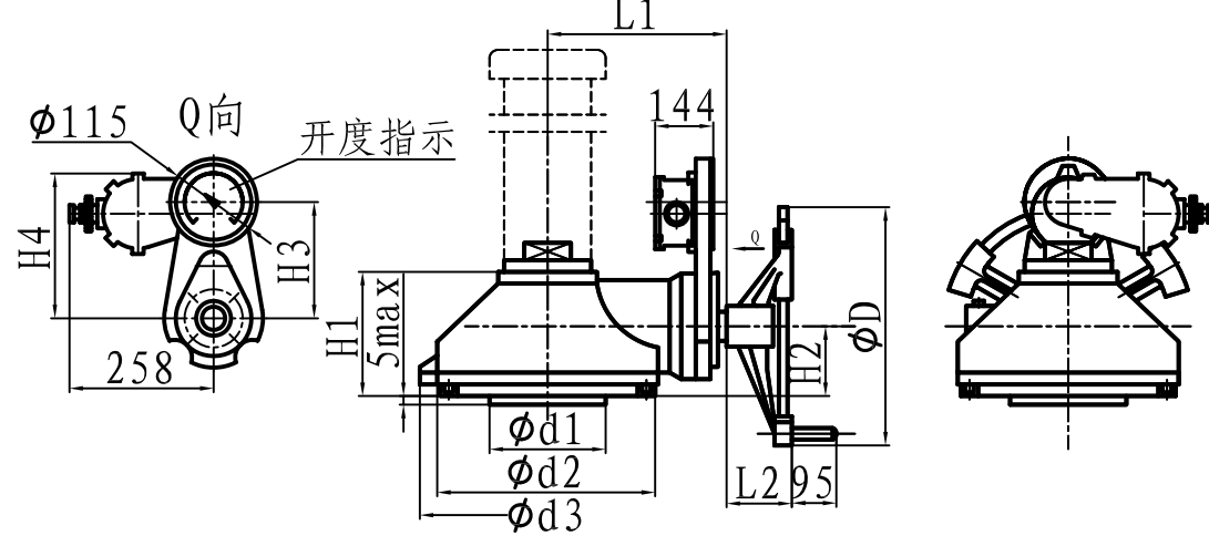
BA-S (带开度指示及微动开关) 外形尺寸
